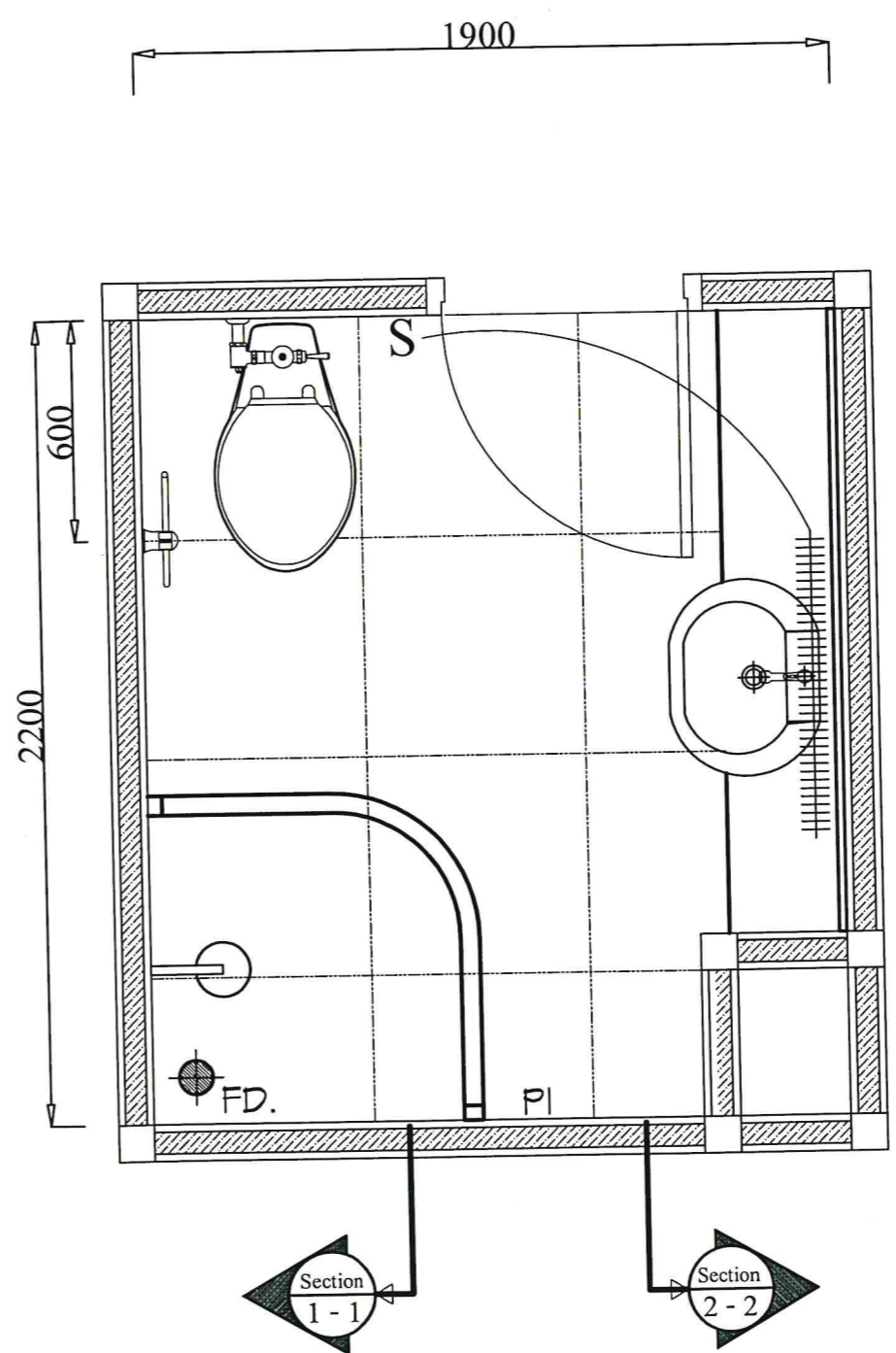
แบบแปลนห้องน้ำ มาตราส่วน 1:100
