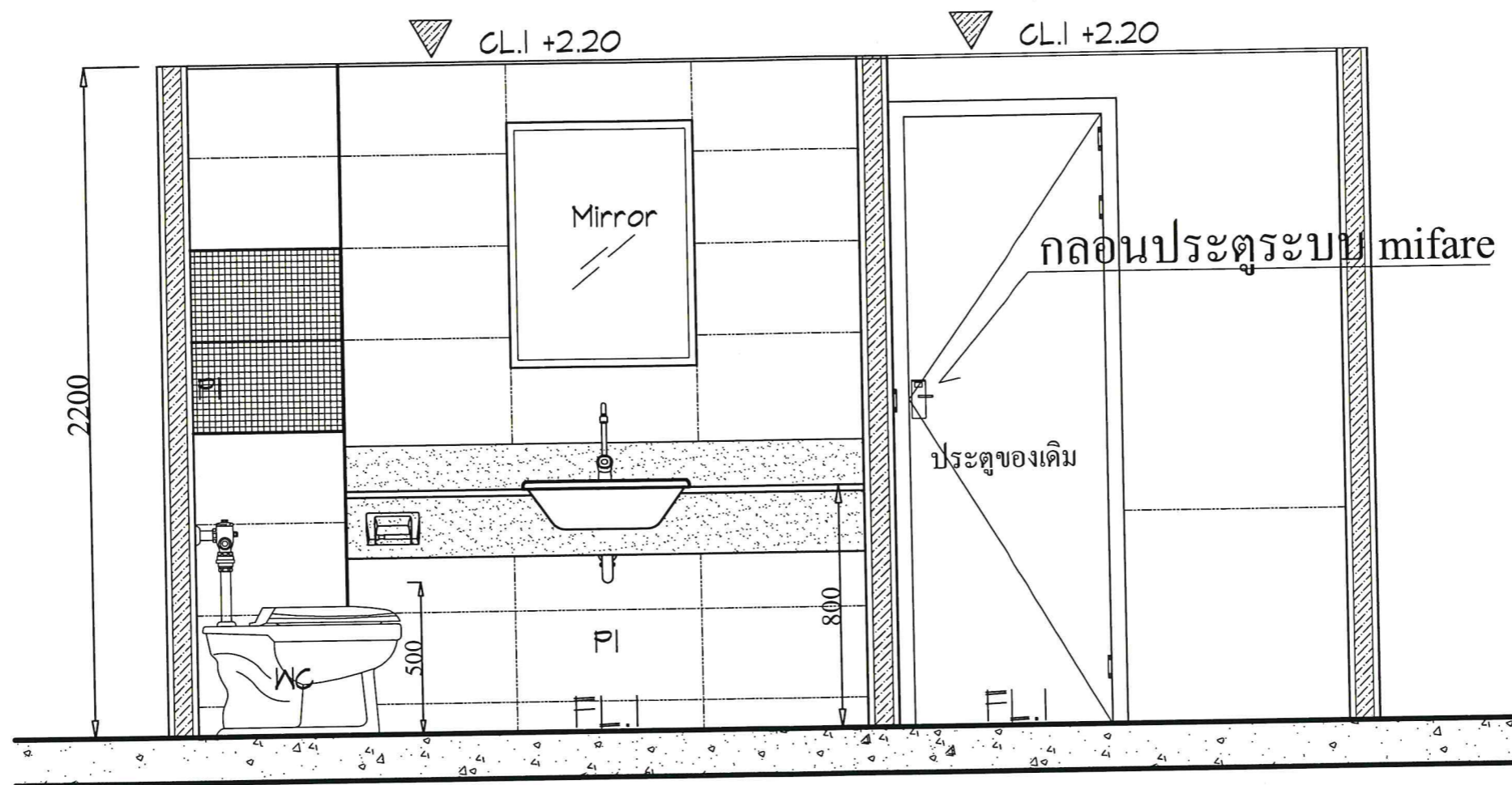
รูปตัด 1-1
