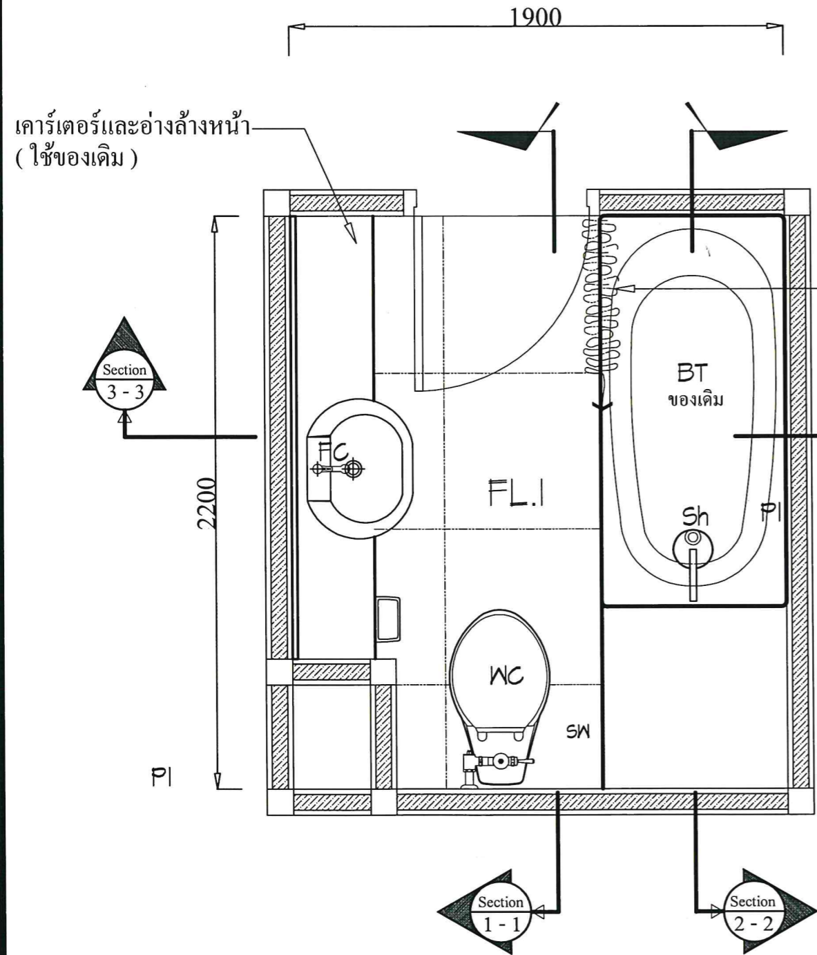
แบบแปลนห้องน้ำชั้น 6
