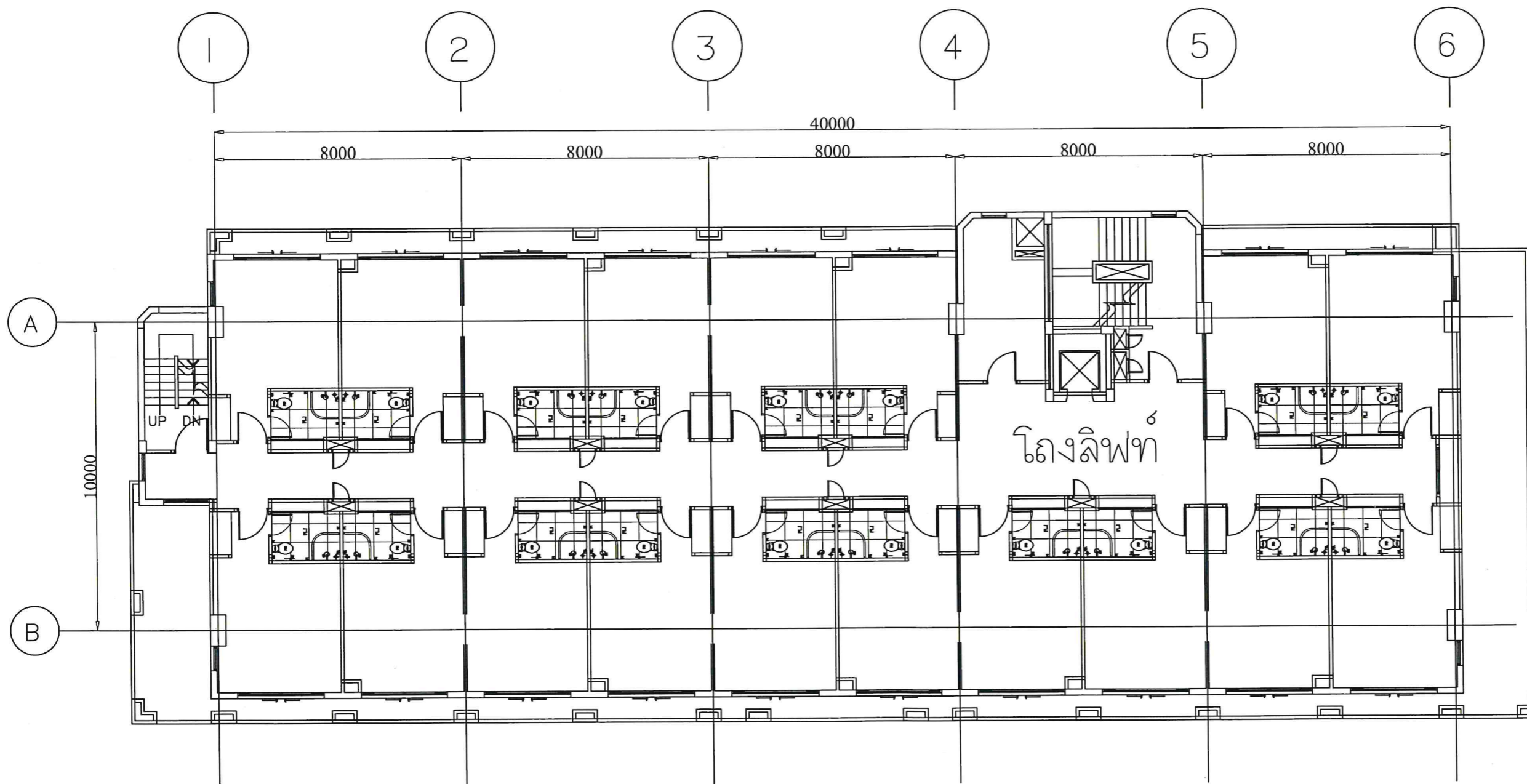
แบบแปลนพื้นที่ชั้นที่ 4-5
