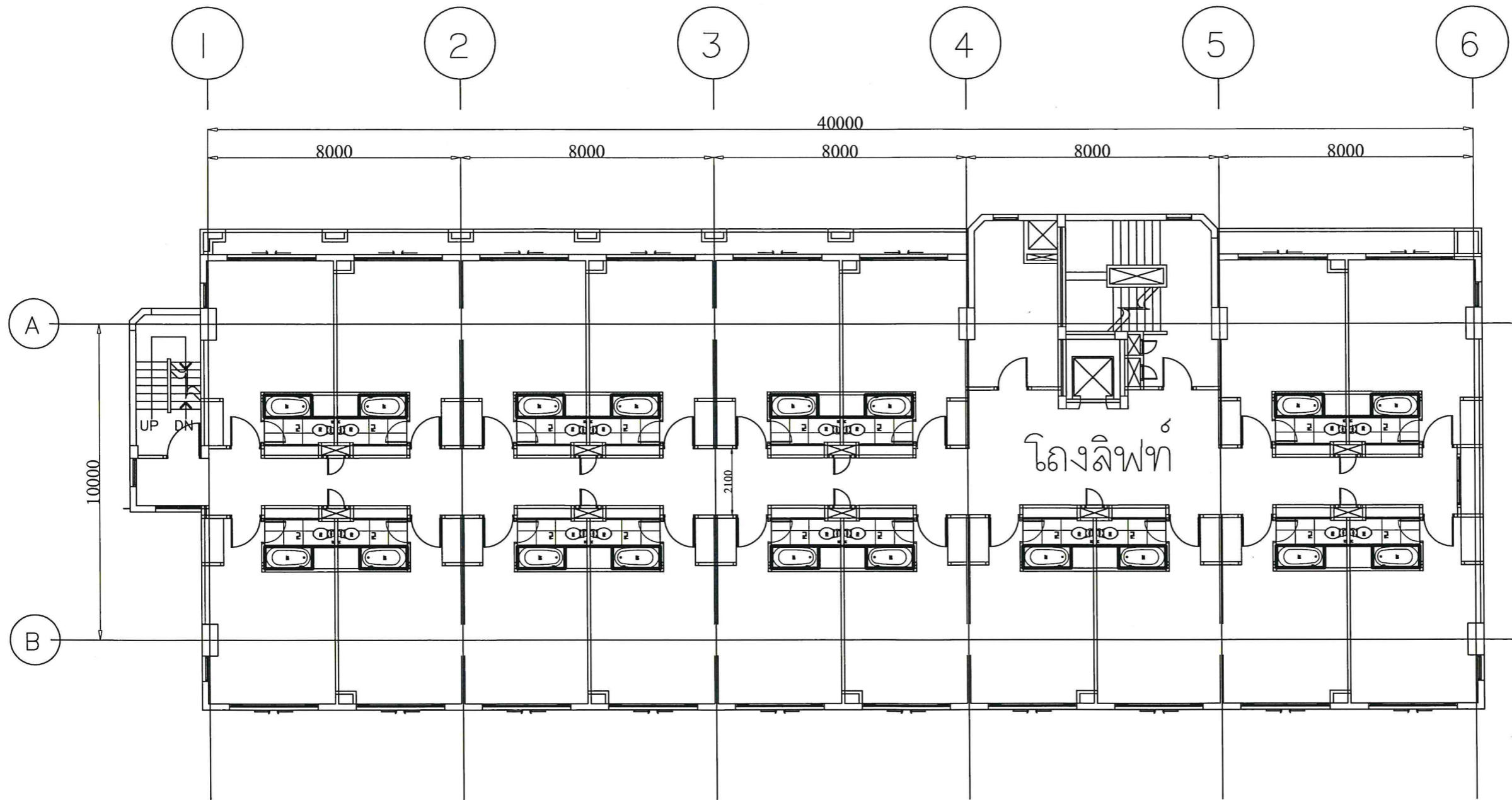
แบบแปลนพื้นที่ 6 มาตรฐาน 1:100 0 0.5 1 2 5
